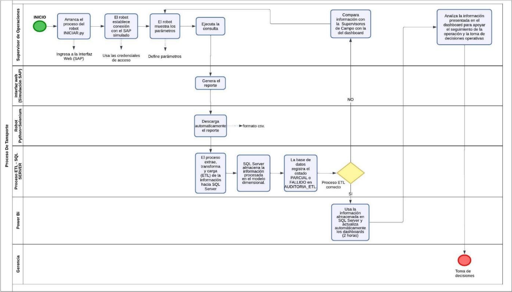
Flujo operativo propuesto (TO-BE) del proceso de Transporte.
